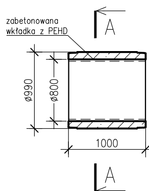
PRZEKRÓJ B-B
