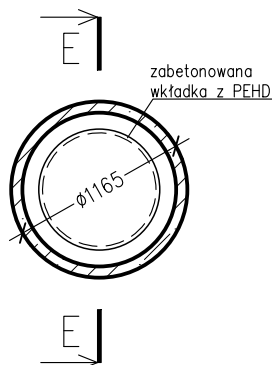
PRZEKRÓJ C-C
